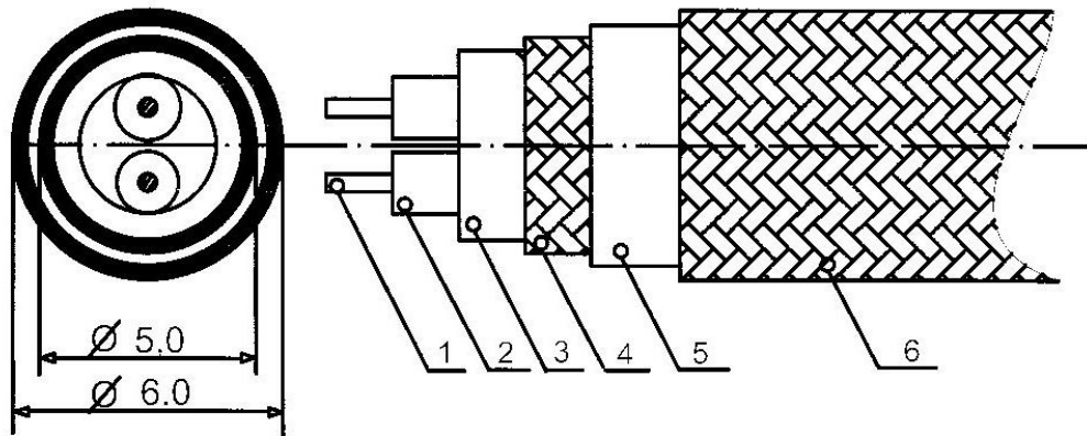
Кабель измерительный жаростойкий экранированный в панцирной броне, двухжильный КИЖЭПн 2х0,4
