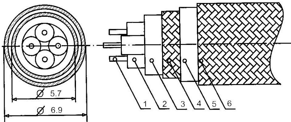
Кабель измерительный жаростойкий экранированный в панцирной броне, четырехжильный
